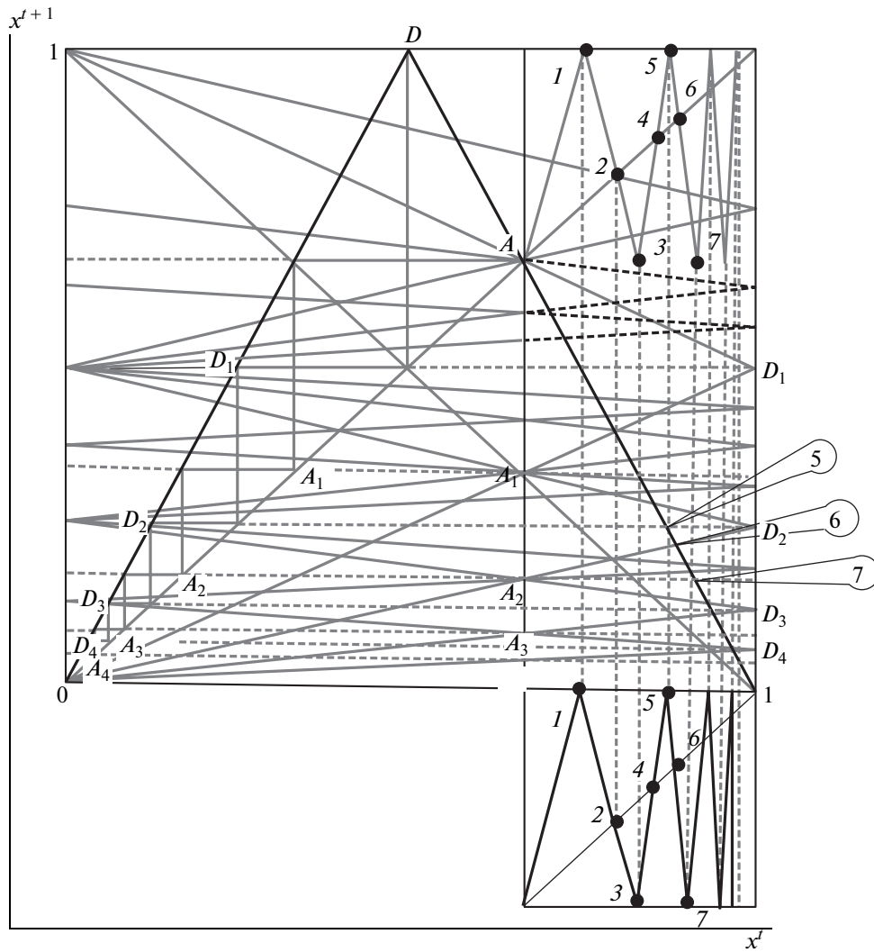
Рис. 4. Графическое представление треугольного отображения, его ЛВн и ОПР (ОПР – вынесенный квадрат в правом нижнем углу и квадрат в правом верхнем углу), а также его n -кратные отображения, повернутые на 90^\circ . ЛВн – сформировано соответствующими фрагментами этих отображений, а ОПР в правом верхнем углу построено из фрагментов исходных n -кратных отображений. Точки, обозначенные цифрами, совпадают с точками рис. 3.
