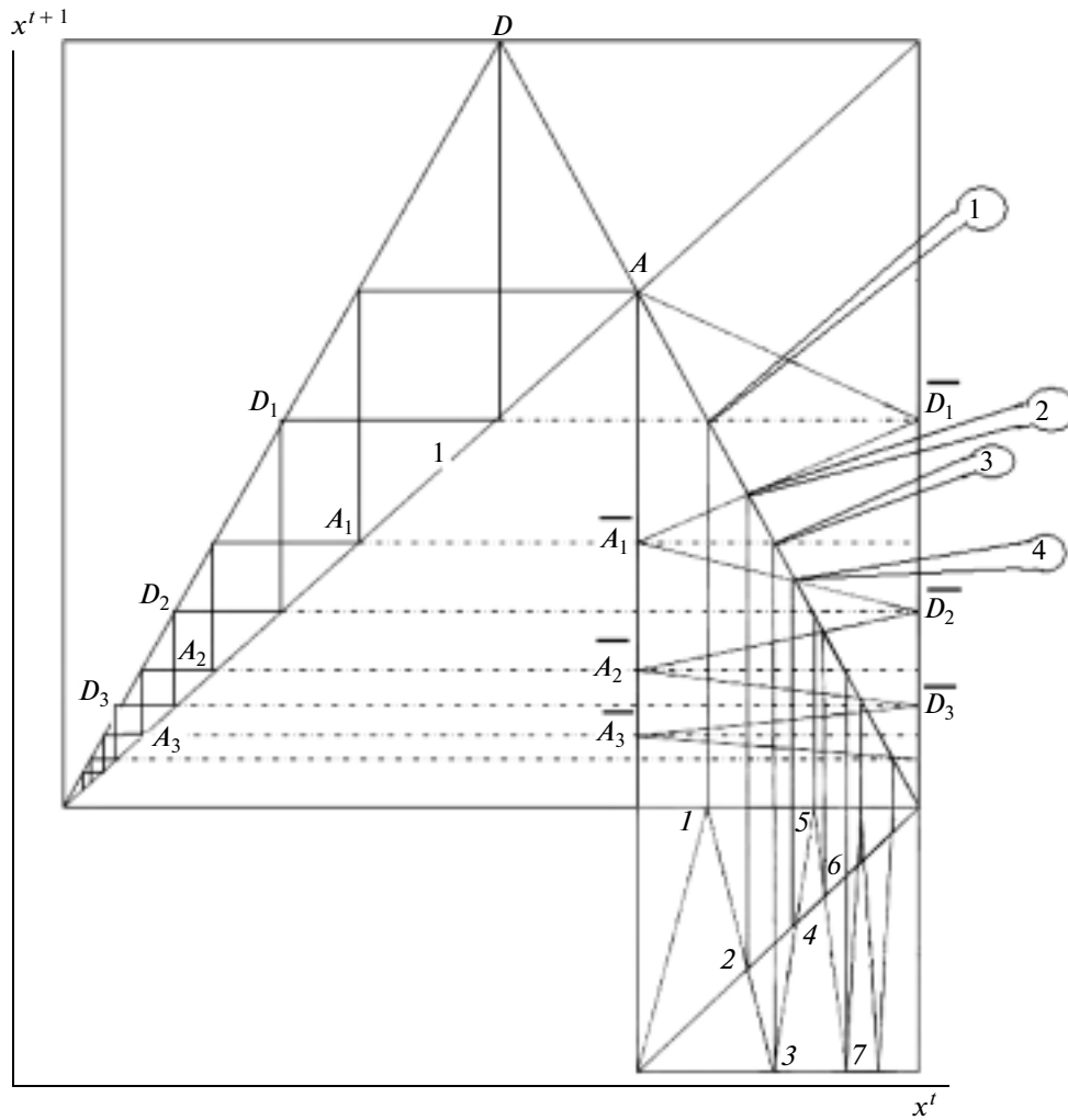
Рис. 3. Графическое представление треугольного отображения, его ЛВn – \bar{A} \bar{D}_1 \bar{A}_1 \bar{D}_2 \bar{A}_2 \bar{D}_3 \bar{A}_3 и ОПР (вынесенный квадрат в правом нижнем углу). Точки 1 и 5 порождены прообразами точки D , точки 3 и 7 порождены прообразами положения равновесия A , точки 2, 4, 6 порождены пересечением графика треугольного отображения с ЛВn и определяют периодические траектории (первая – периода 2, две другие – периода 3).
