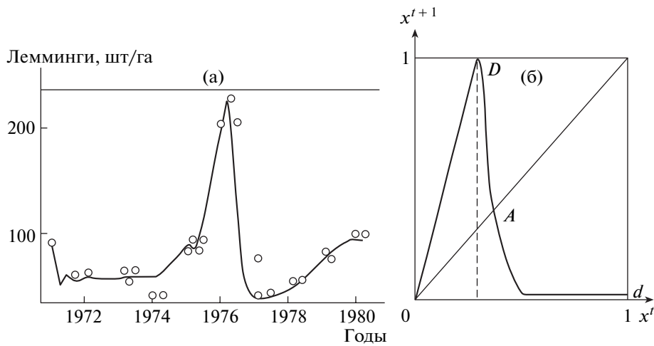
Рис. 1. а – расчетная динамика популяции леммингов (по результатам одного из имитационных экспериментов с моделью растительность–лемминги–песцы (сплошная кривая) и зарегистрированная на острове Врангеля динамика изменения численности копытного лемминга (кружки) [6]. б – Графическое представление разностного уравнения X^{t+1} = F(X^t) , связывающего нормированные численности леммингов X^t в двух соседних годах, основанные на анализе моделей тундровых популяций и сообществ. Здесь D – точка достижения максимального значения численности, A – равновесная численность, d – численность леммингов в оптимальном биотопе (понятие “оптимальный биотоп” было введено в работах [3, 5] и подразумевает область пространства обитания с оптимальными условиями проживания; в оптимальном биотопе при любых условиях выживает определенная численность зверьков).
