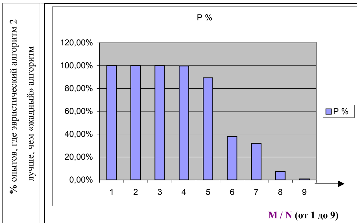
Рис. 4. Результаты ряда экспериментов с эвристическим алгоритмом 2
