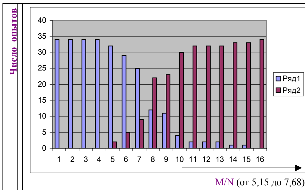
Рис. 3. Результаты ряда экспериментов с эвристическим алгоритмом 1
