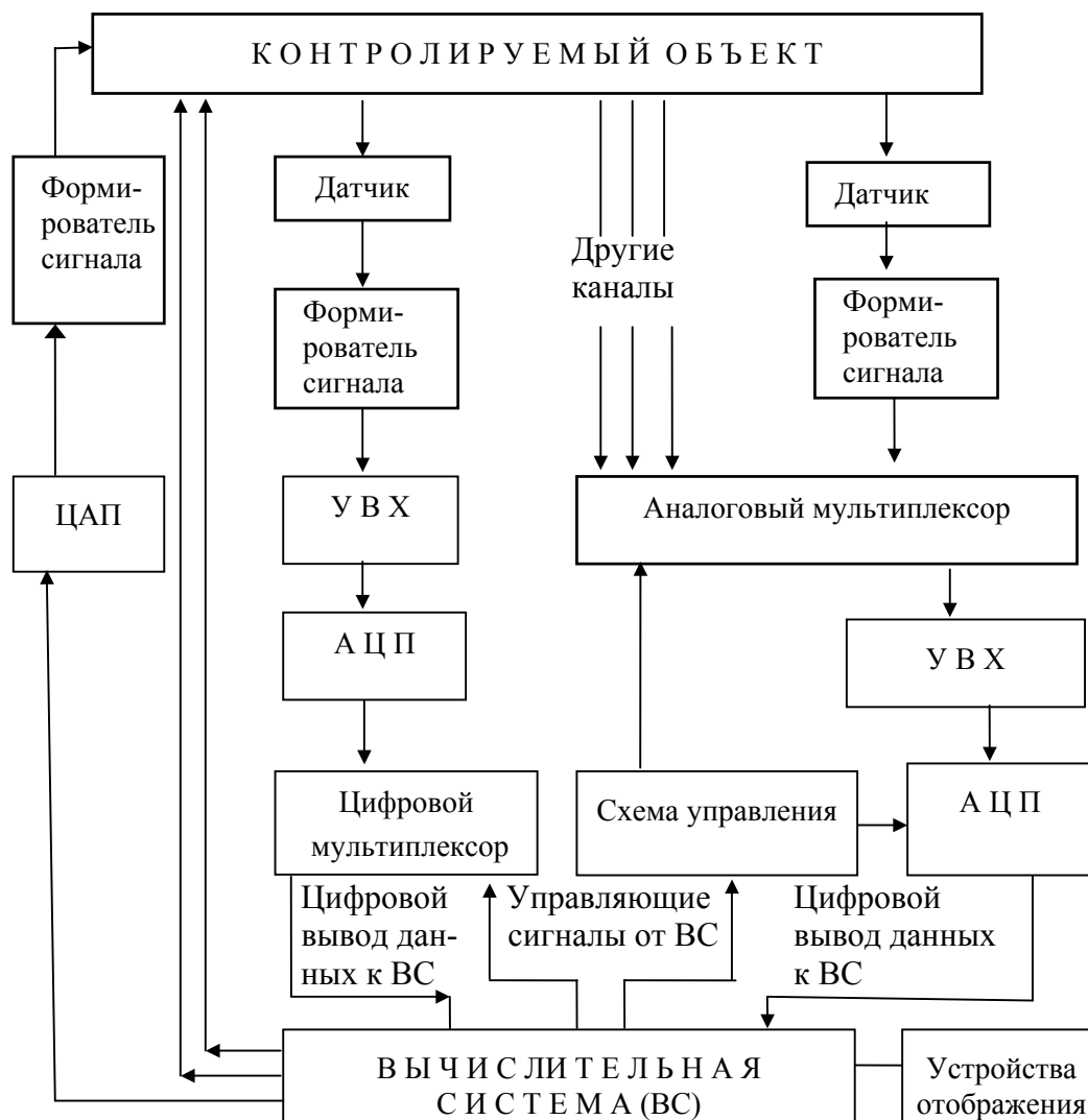
Рис. 1. Схема использования ЭВМ для управления физическими процессами. Потoki информации и аппаратные средства типичной многоканальной системы сбора данных и управления представляются на различных устройствах отображения (дисплеях и т.п.) и, кроме того, если необходимо, вырабатываются управляющие воздействия, которые после соответствующих преобразований поступают к объекту, управляя его функционированием. АЦП – аналогово-цифровой преобразователь. ЦАП – цифро-аналоговый преобразователь. УВХ – устройства выборки-хранения аналогового сигнала.
